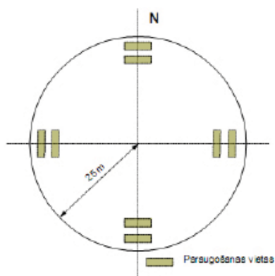
2. attēls. Augsnes paraugu ņemšanas vietu shēma.
