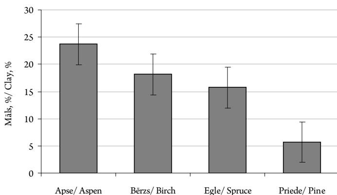
9. attēls. Māla īpatsvars minerālaugsnēs 40...80 cm dziļumā mežaudzēs ar dažādām valdošajām koku sugām. Figure 9. Share of clay particles in mineral soils at 40...80 cm depth in forest stands with different dominant species.
