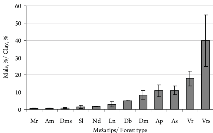
8. attēls. Māla saturs dažādu meža tipu minerālaugsnēs 40...80 cm dziļumā.
