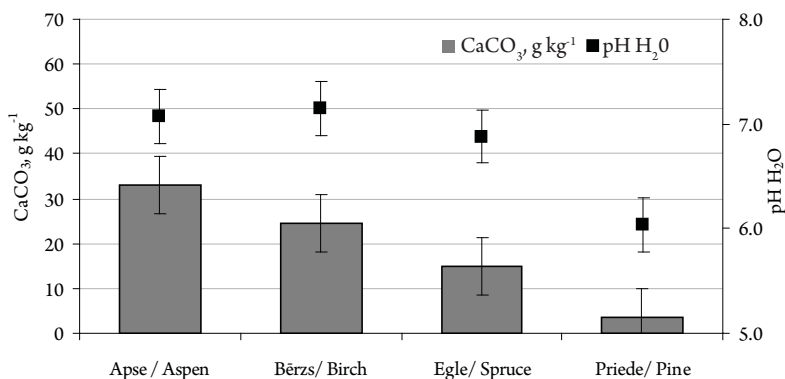
3. attēls. Sakarība starp \text{CaCO}_3 saturu un \text{pH H}_2\text{O} augsnē 40...80 cm dziļumā.
