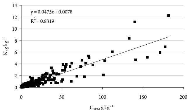
4. attēls. Sakarība starp kopējo slāpekli un organisko oglekli minerālaugsnēs ( C_{\text{org.}} < 200 \text{ g kg}^{-1} ).
