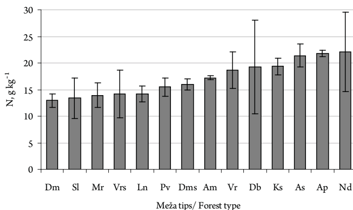
6. attēls. N_{kop.} saturs dažādos meža tipos O horizontā.
