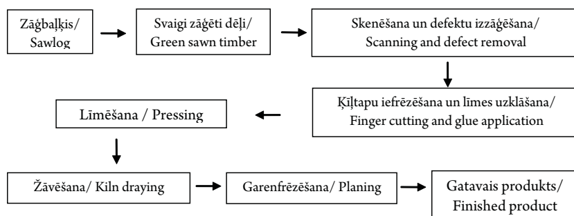
1. attēls. Produktu izgatavošanas principiālā shēma, izmantojot paaugstināta mitruma koksnes līmēšanas tehnoloģiju.
