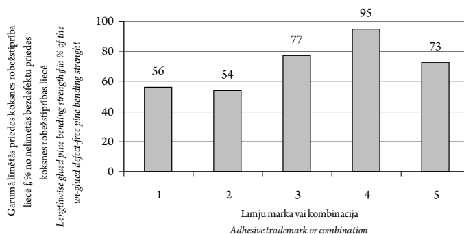
2. attēls. Garumā līmētas priedes koksnes robežstiprība liecē % no nelīmētas, bezdefektu priedes koksnes robežstiprības liecē.
