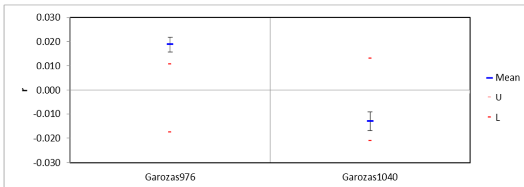
4.3. attēls. Savstarpējā radniecība katrā sēkļu partijā un salīdzinājums ar sagaidāmajām 95% robežām, analizējot visas partijas kopā.
