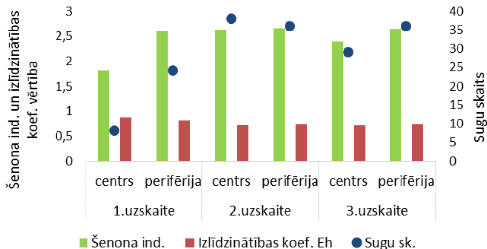
14. attēls. Putnu sugu daudzveidības salīdzinājums 200 m rādiusā ap dabā novērotiem riestojošajiem medņu gaiļiem (centra teritorija) un pārējās stacionāro uzskaišu teritorijās 1 km rādiusā ap ģeometriskiem riestu centriem (perifērā teritorija).
