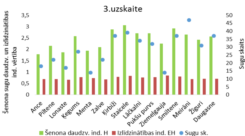
12. attēls. Putnu sugu daudzveidība medņu riestos, atkārtojot uzskaiti 3 reizes – pirms riesta perioda, medņu riestošanas un ligzdošanas periodā, un pēc ligzdošanas perioda.
