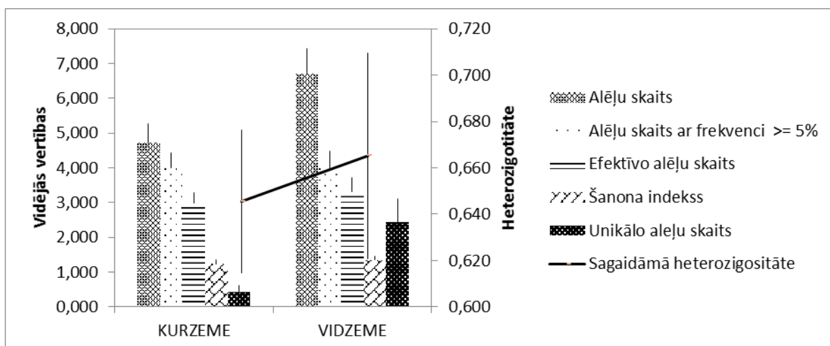
17. attēls. Ģenētiskās daudzveidības rādītāju salīdzinājums starp Kurzemes un Vidzemes mikropopulācijām.
