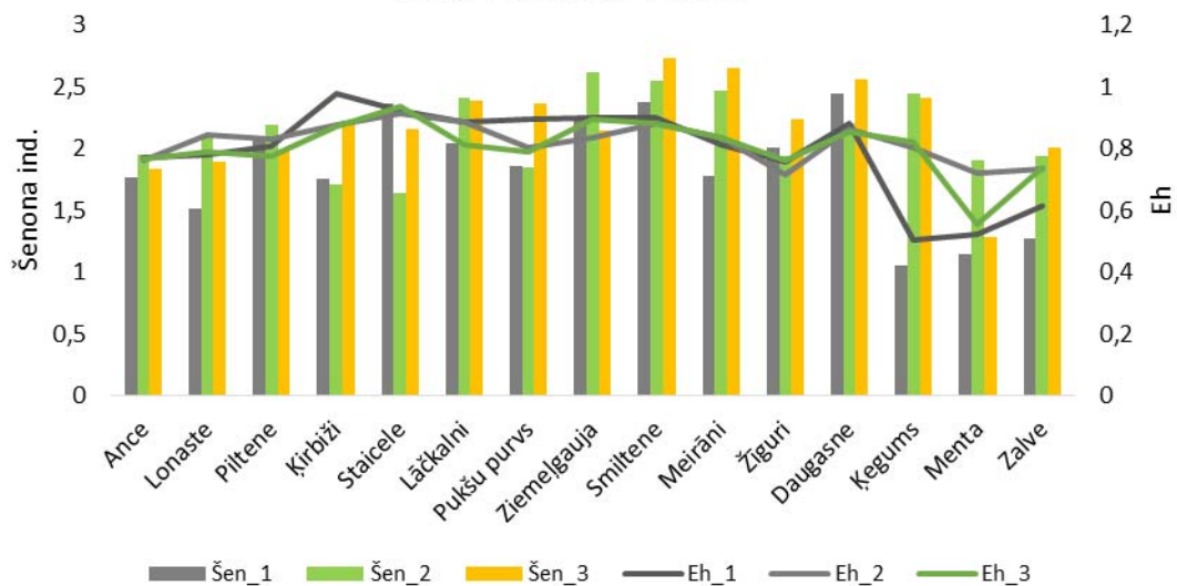
Šenona daudzveidības un izlīdzinātības indeksi riestos visās uzskaites reizēs
