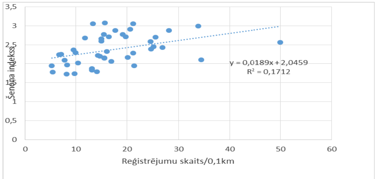
16. attēls. Putnu sugu Šenona daudzveidības indeksa atkarība no reģistrētā visu sugu indivīdu kopējā blīvuma. Pīrsona korelācija: r = 0,414 , p = 0,005 , n = 44 .
